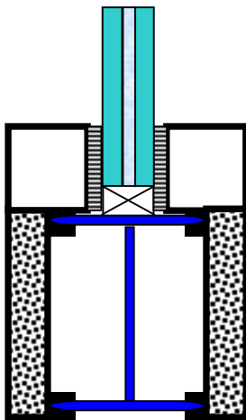
System Jansen Janisol thermisch getrennt symmetrisch
